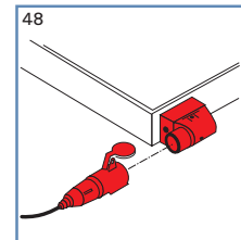
48 Steckdose für Tasterkabel oder Zuleitung am Rahmen montiert, mit Stecker am Kabel 49 Steuerspannung 24 V AC = serienmäßig
