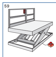
58 Fußtaster mit Not-Aus-Taster in Tischplatte eingelassen, Not-Aus-Taster lose an 3 m Kabel anstatt Handtaster, Geländer 1 m erforderlich 59 Handtaster mit Not-Aus-Taster am Geländer, Not-Aus-Taster lose an 3 m Kabel anstatt Handtaster
