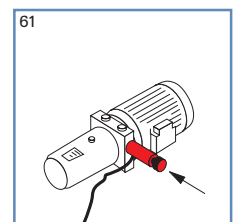
60 Hydraulikaggregat und Steuerung 2 m außerhalb in einer Leckölwanne 61 Notablass am Aggregat (Sperventile am Zylinder entfallen)
