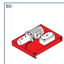
60 Hydraulikaggregat und Steuerung 2 m außerhalb in einer Leckölwanne 61 Notablass am Aggregat (Sperventile am Zylinder entfallen)
