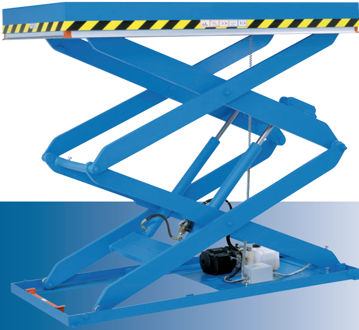
Hubtisch ELD 1-26-9
