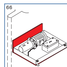
66 Aggregat außerhalb mit 5 m Schlauch, Leckölwanne und Wandkonsole
